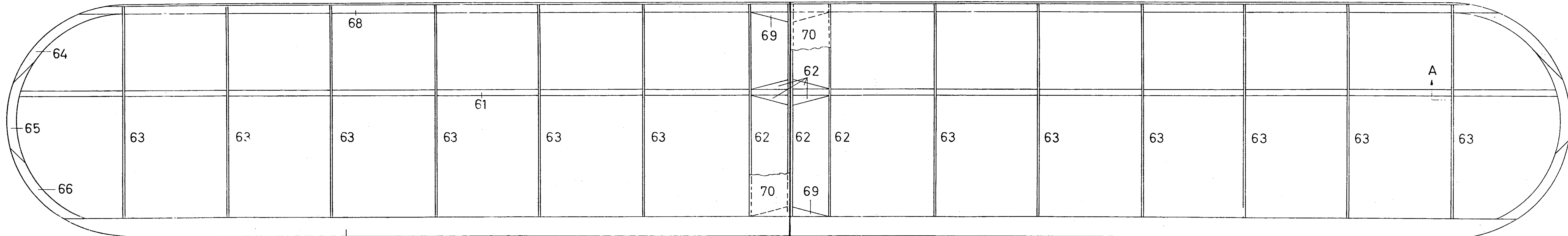
Der Tragflügel ist ohne V-Form gestreckt dargestellt. The wing is shown flat, i.e. actual size.
