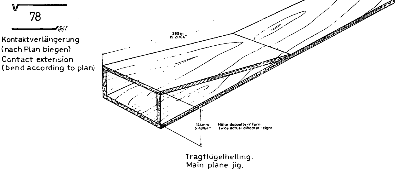
Der Tragflügel ist ohne V-Form gestreckt dargestellt. The wing is shown flat, i.e. actual size.
